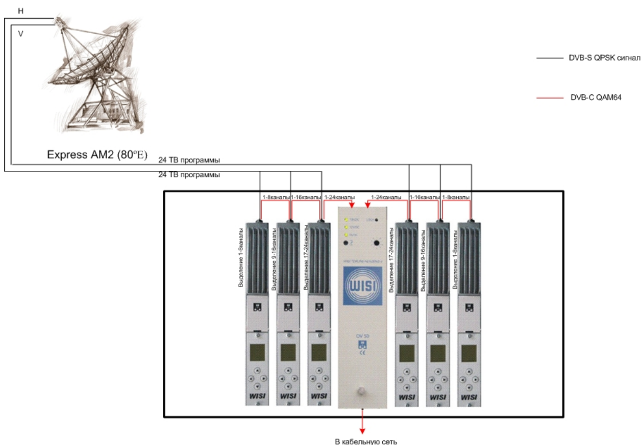
Рис.2 Головная станция WISI OV50A
